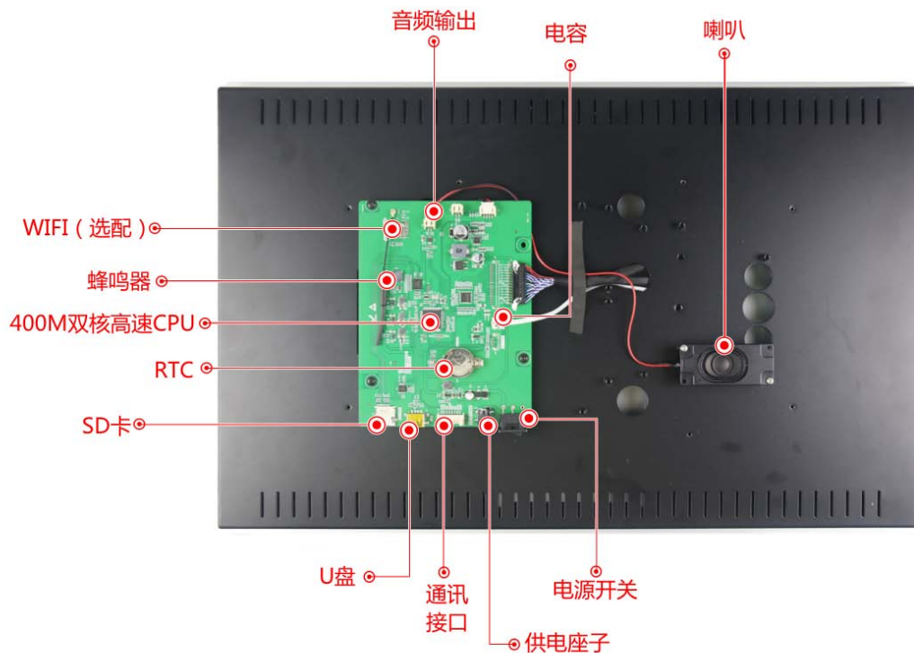
图 1-2 硬件配置图
