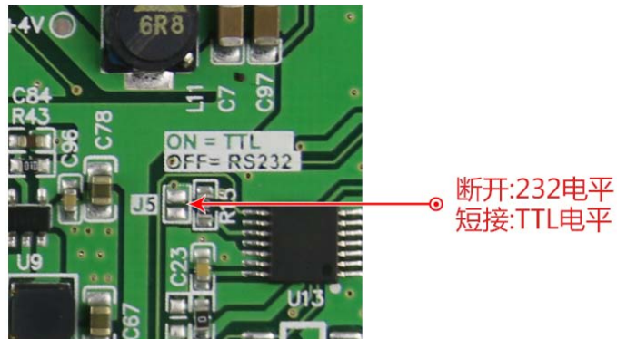
图 7-1 RS232 和 TTL 转换示意图
